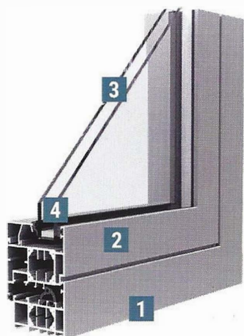
Špecifikácia obrázku: 1 - rám č. K518611X ST, 2 - krídlo č. K518712X ST, 3 - dvojsklo 4 - teplý rámček Swisspacer
