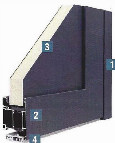
Špecifikácia obrázku: 1 - rám č. K518731X ST, 2 - krídlo č. K518746X ST, 3 - výplň hrúbky 44mm 4 - nízky prah
