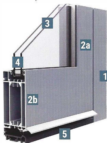
Špecifikácia obrázku: 1 - rám č. K518106X, 2a - krídlo č. K518115X, 2b - okop č. K518103X, 3 - dvojsklo 4 - teplý rámček Swisspacer 5 - nízky prah
