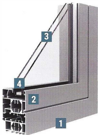
Špecifikácia obrázku: 1 - rám č. K518101X, 2 - krídlo č. K518332X, 3 - dvojsklo 4 - teplý rámček Swisspacer
