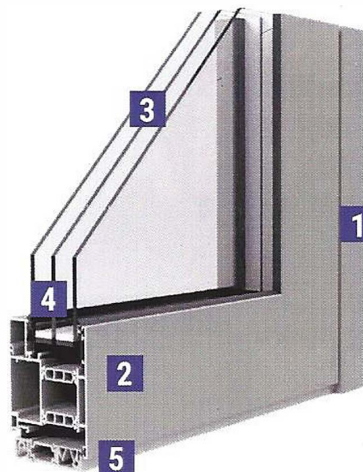
Špecifikácia obrázku: 1 - rám č. SP814 2 - krídlo č. SP825 3 - trojsklo 4 - teplý rámček Swisspacer 5 - nízky prah
