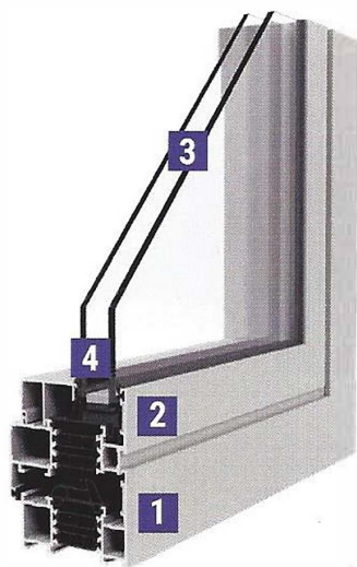
Špecifikácia obrázku: 1 - rám č. SP011 2 - krídlo č. SP021 3 - dvojsklo 4 - teplý rámček Swisspacer
